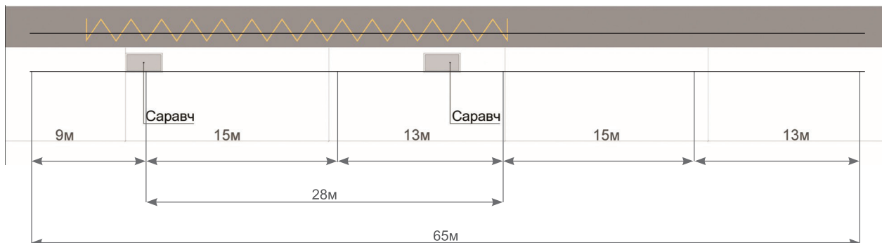
Зураг 14. Залгаа автобус зогсох талбай (Жишээ зураг)
