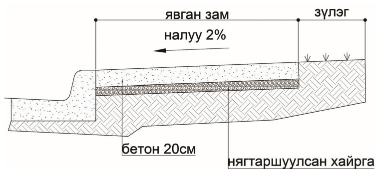
Зураг 19. Зорчих хэсэг явган замтай уялдах ерөнхий схем-2
