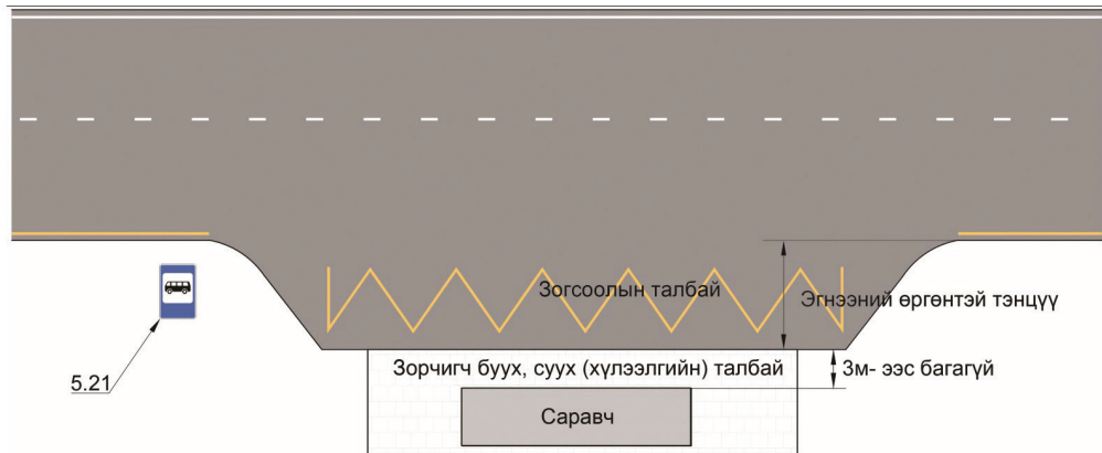
5.2.1. Тэмдэг «Автобусны зогсоол» (Жишээ зураг)
