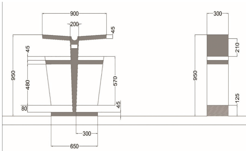
Зураг 31. Автобусны зогсоолын хогийн савны хэмжээ (мм), загвар (Жишээ зураг)
