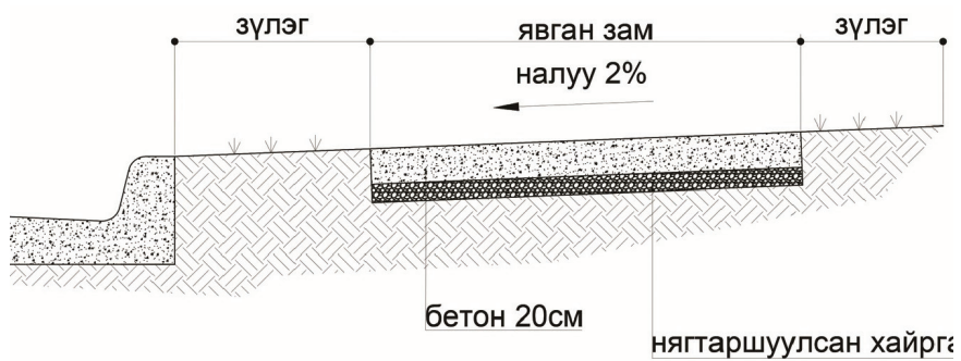
Зураг 18. Зорчих хэсэг явган замтай уялдах ерөнхий схем-1
