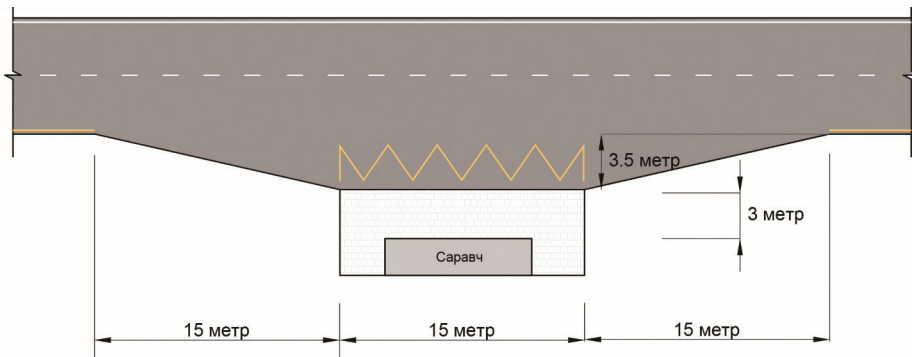
Зураг 3. 3-р зэрэглэлийн зогсоолын зай хэмжээ (Жишээ зураг)
