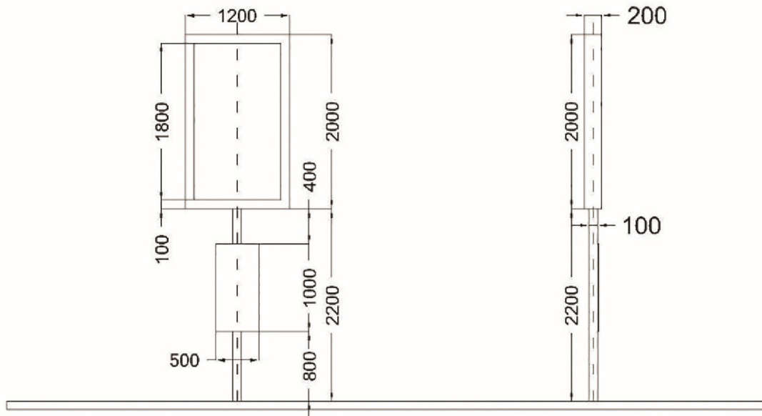
Зураг 27. Мэдээллийн самбарын хэмжээ (Жишээ зураг)
