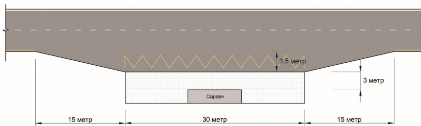
Зураг 2. 2-р зэрэглэлийн зогсоолын зай хэмжээ (Жишээ зураг)
