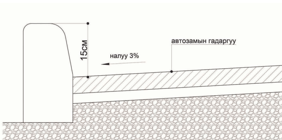
Зураг 17. Зорчих хэсгийн хийц бүтээцийн ерөнхий схем
