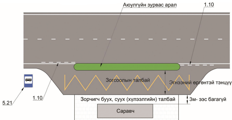
Зураг 4. Зогсоолын талбайг аюулгүйн зурвас арлаар тусгаарласан байдал. (Жишээ зураг)
